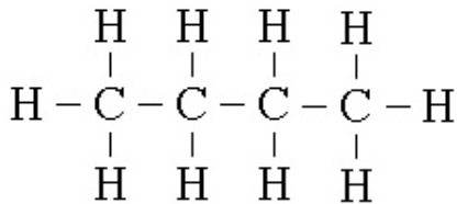
butano (C 4 H 10 )
