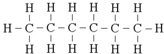
esano (C 6 H 14 )
