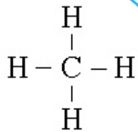
metano (CH 4 )
